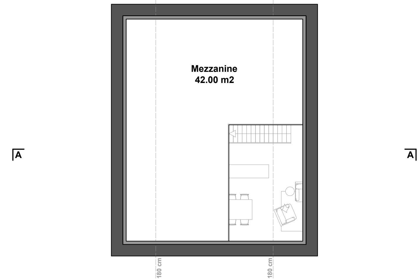
Combles - 1:100 - Configuration 2 appartements
