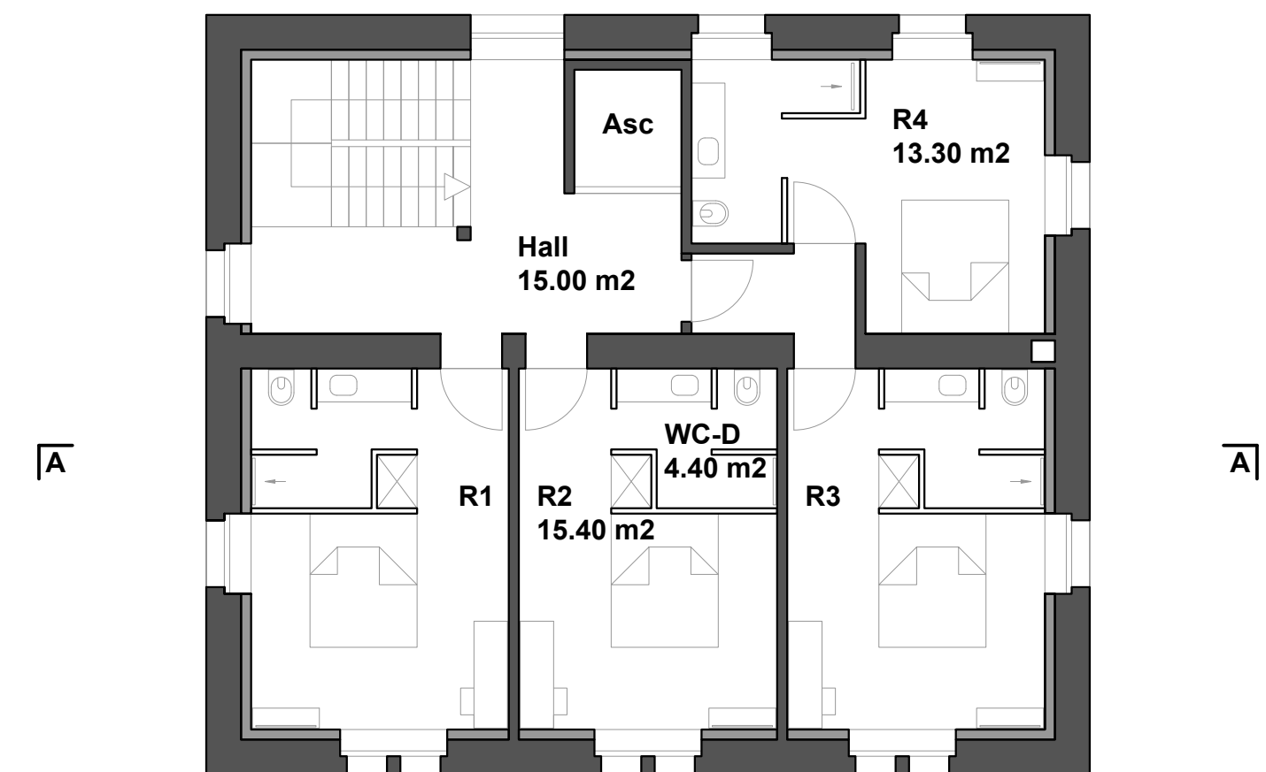
Etage - 1:100
