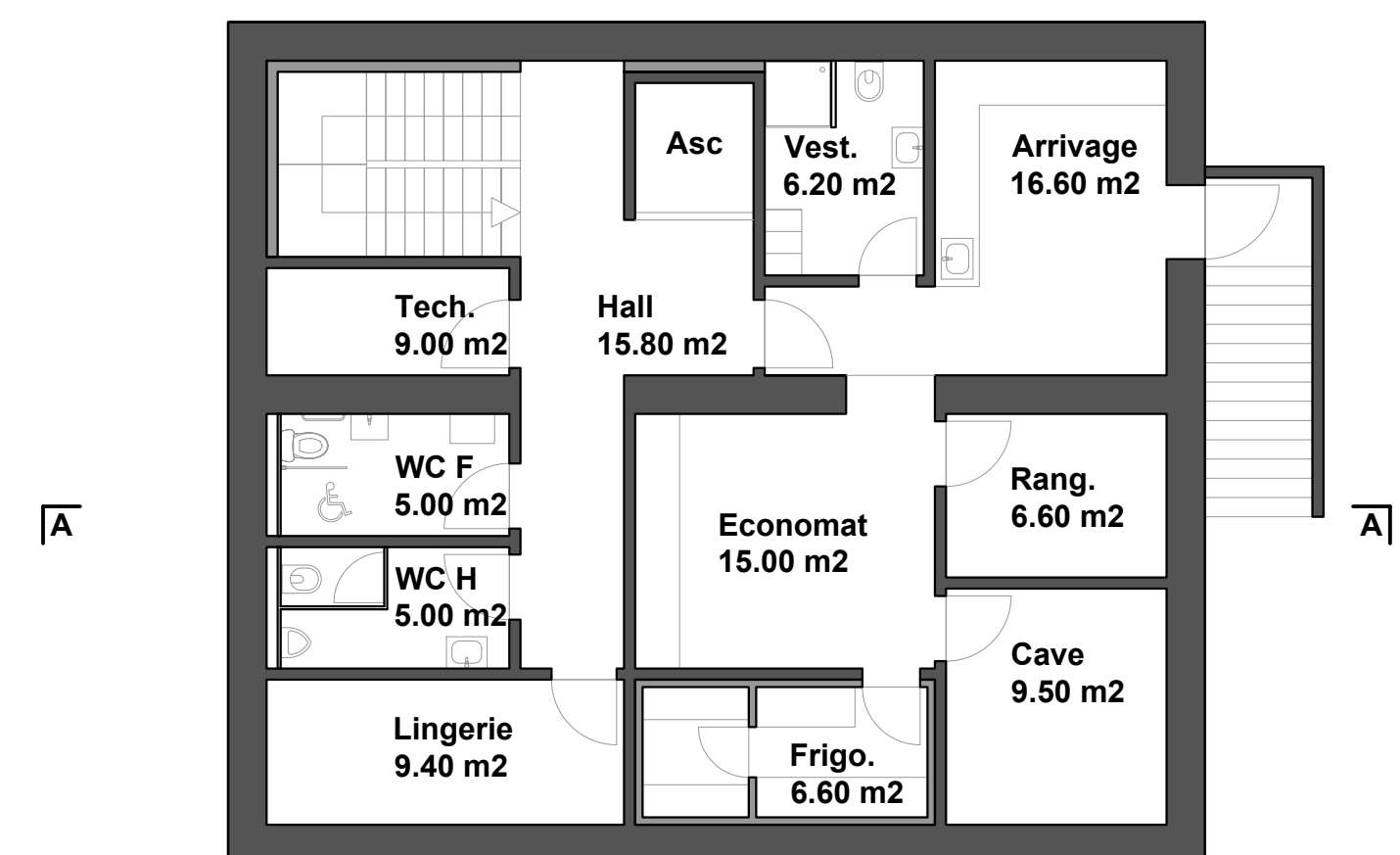
Sous-sol - 1:100
